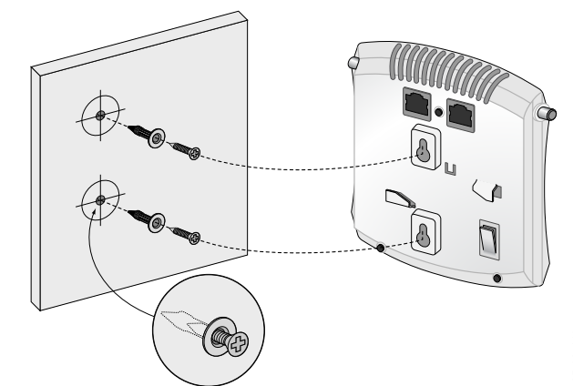
Gambar 4 Memasang Titik Akses Seri W-AP90 di Dinding
